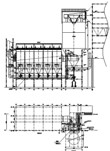
B-B 反应塔处上行管道立面布置
